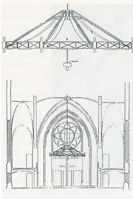
Lüster-Entwurf
